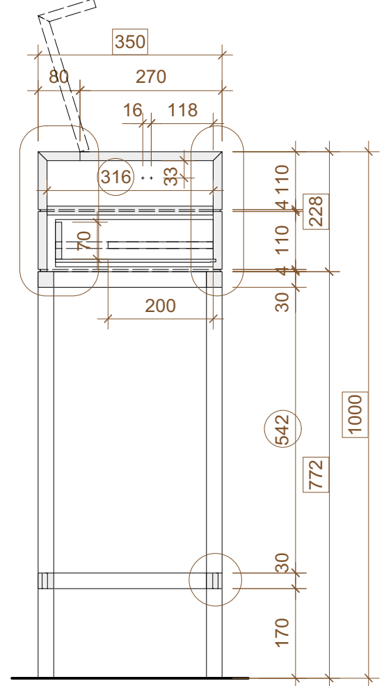
SCHNITT / COUPE C-C
