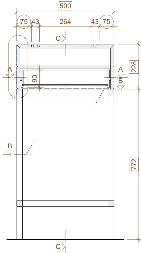
SCHNITT / COUPE D-D
